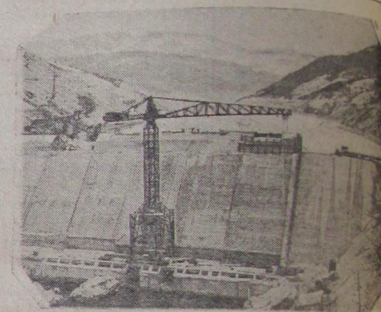
ნიმერკაპკაბაძის ოლქი. ტერებლია-რიკის ჰიდროელსადგურის მძღვრმა კაშალა გზა გადაუღობა მდინარე ტერებლს. იგეგმა წყალსაცავი, უმოკლეს დროში გვირახებით და მილსადენებით 200 მეტრის სიმაღლიდან წყალი წავა ტურბინებში. მალე ჰესი ელექტროენერჯიას მისცემს სამრეწველო საწარმოებს, რკინიგზის ტრანსპორტსა და ოლქის კომუნისტურებს. სურათზე: ტერებლია-რიკის ჰესის კაშხალი გზას უღობავს მდინარე ტერებლს.
