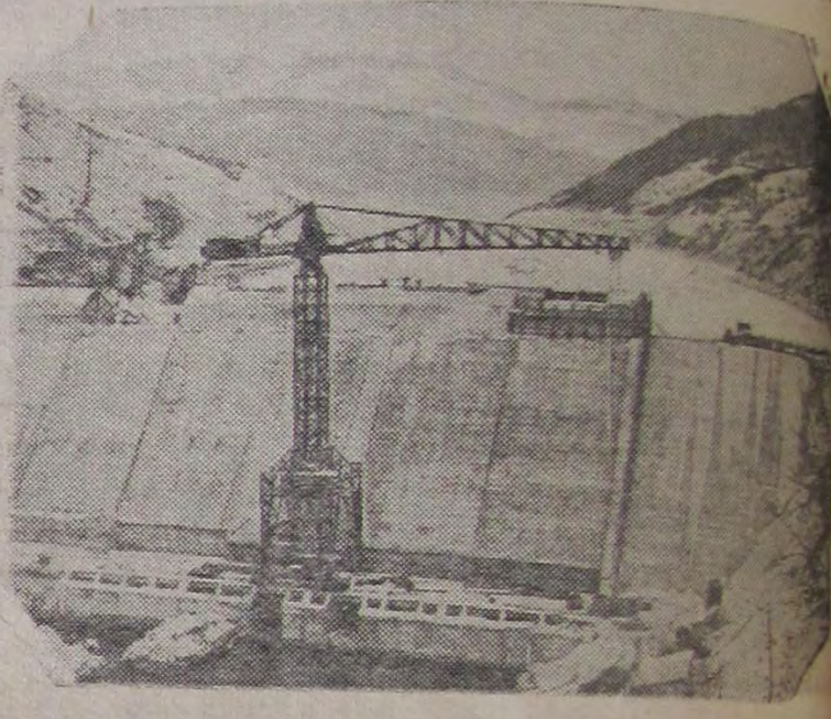
იმერკაპკატების ოლქი. ტერებლია-რიკის ჰიდროელსადგურის მძლავრმა კაშხალმა გზა გადაუღობა მდინარე ტერებლს, იცვება წყალსაცავი. უზოკლს დროში გვირბეებით და მილსადენებით 200 მეტრის სიმაღლიდან წყალი წავა ტურბინებში. მალე ჰესი ელექტროენერჯიას მისცემს სამრეწველო საწარმოებს, რკინიგზის ტრანსპორტსა და ოლქის კოლმურნეობებს. სურათზე: ტერებლია-რიკის ჰესის კაშხალი გზას უღობავს მდინარე ტერებლს.
